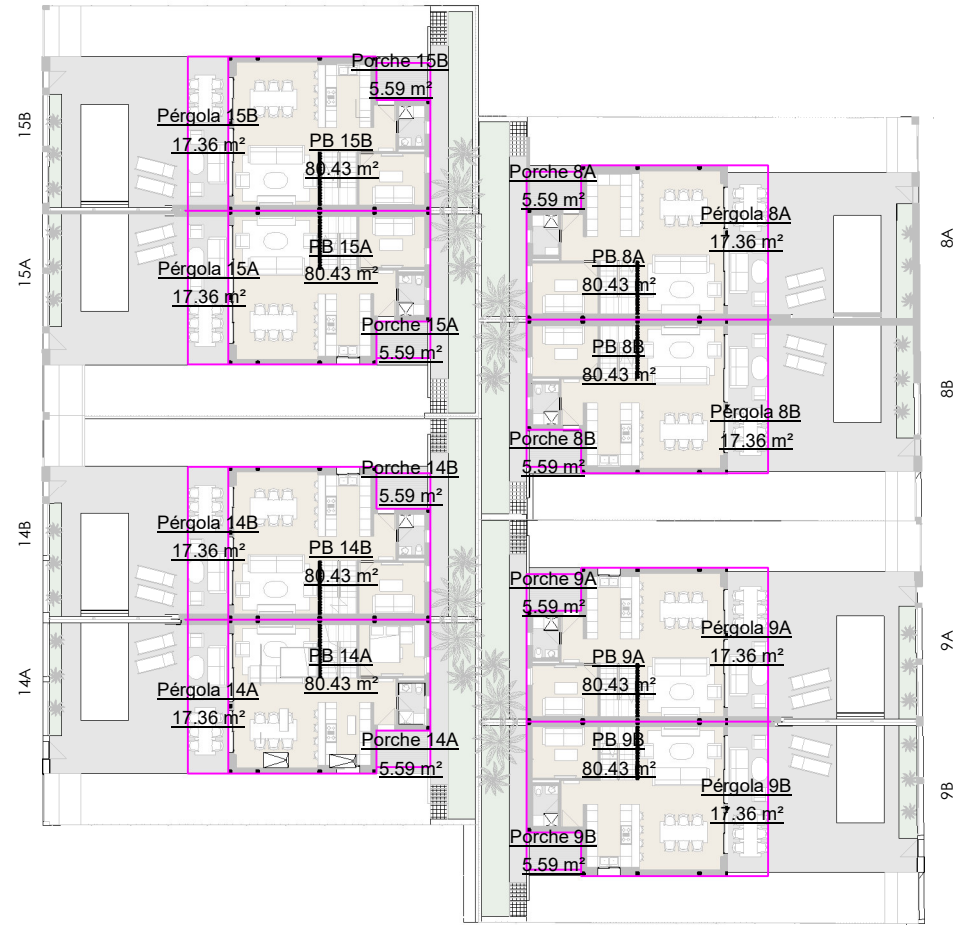
Superficie Construida PB 1 : 400
